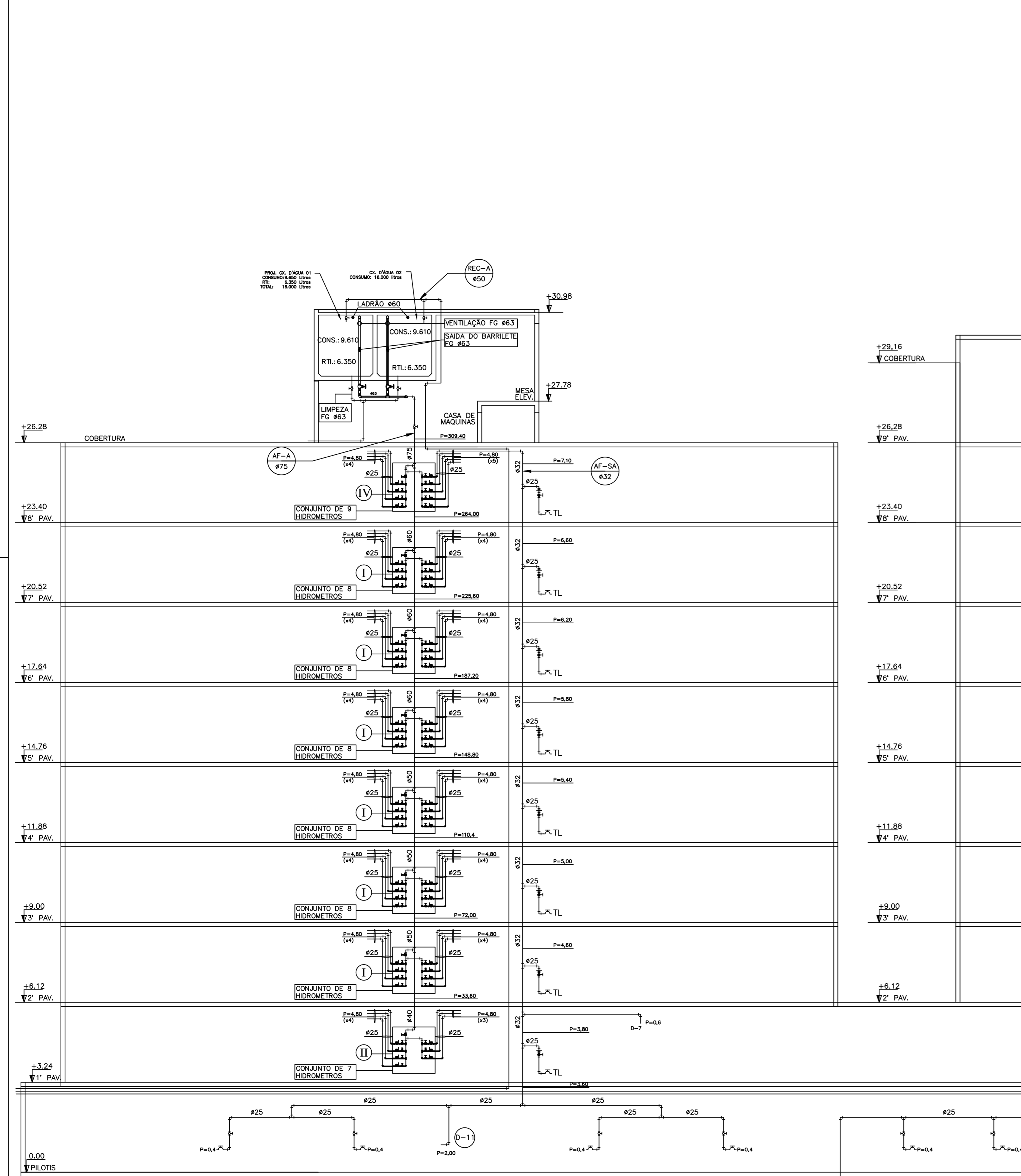
ESQUEMA VERTICAL - BLOCA A SEM ESCALA
