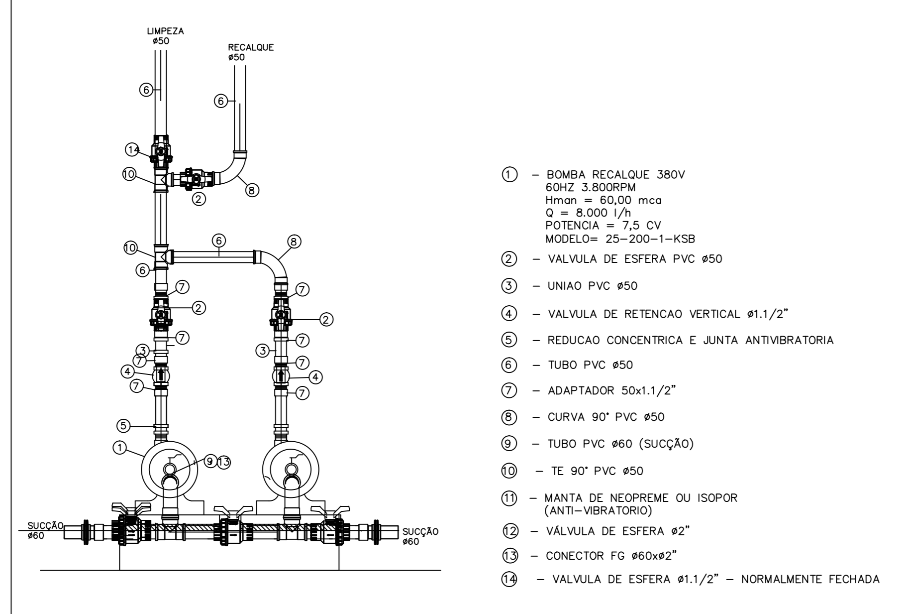
D-B DETALHE DA BOMBA DE RECALQUE COM LIMPEZA SEM ESCALA
