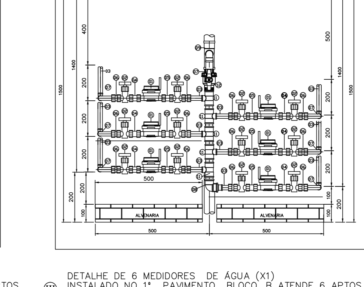
DETALHE DE 6 MEDIDORES DE ÁGUA (X1) INSTALADO NO 1º PAVIMENTO BLOCO B ATENDE 6 APTOS SEM ESCALA
