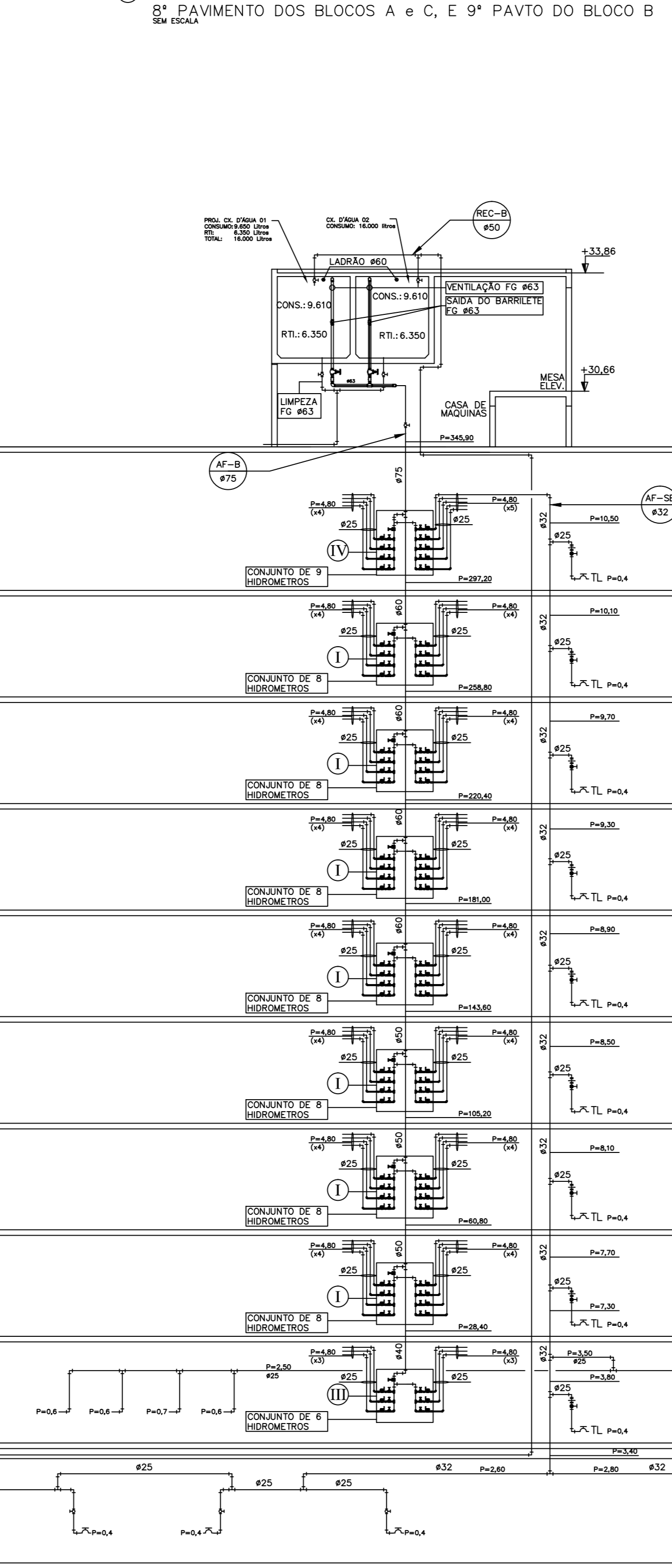
ESQUEMA VERTICAL - BLOCA B SEM ESCALA
