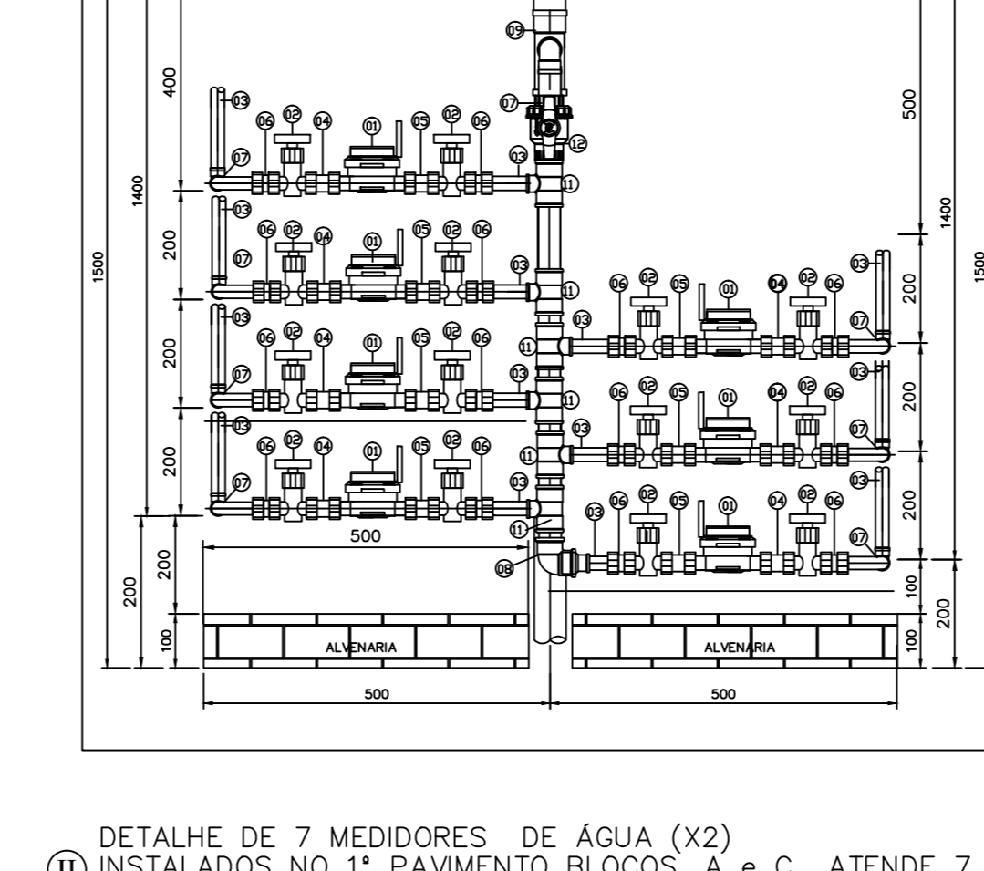
DETALHE DE 7 MEDIDORES DE ÁGUA (X2) INSTALADOS NO 1º PAVIMENTO BLOCOS A e C ATENDE 7 APTOS SEM ESCALA
