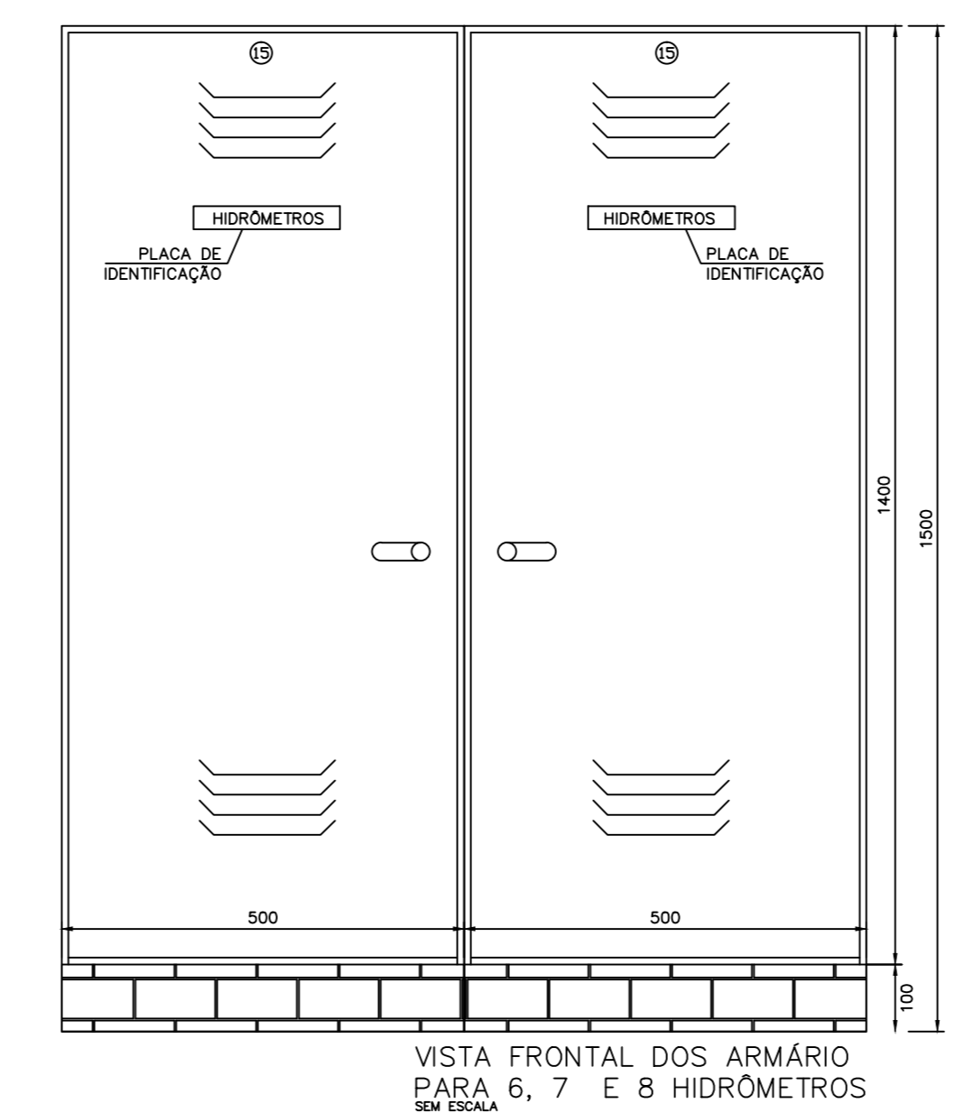
VISTA FRONTAL DOS ARMÁRIOS PARA 6, 7 E 8 HIDRÔMETROS SEM ESCALA
