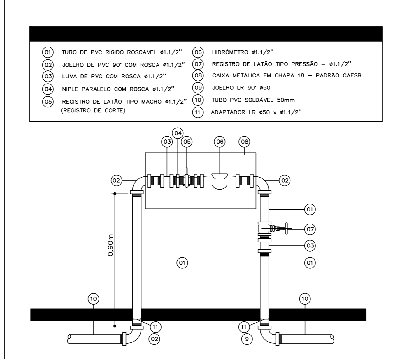
DETALHE HIDRÔMETRO DE ENTRADA SEM ESCALA
