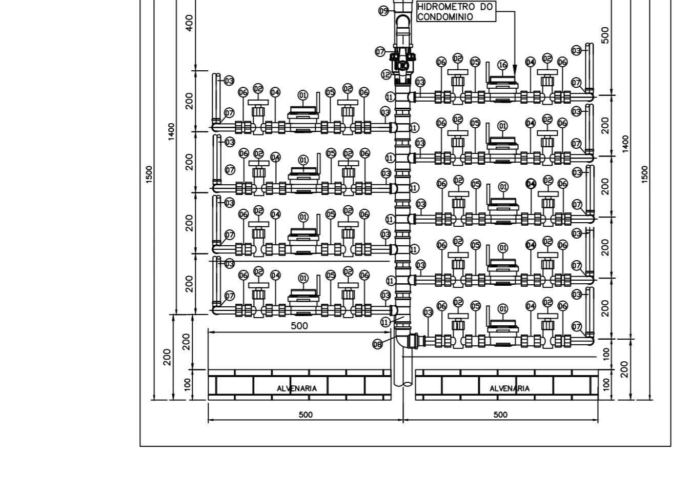
DETALHE DE 9 MEDIDORES DE ÁGUA (X3) INSTALADOS NO ÚLTIMO PAVIMENTO ATENDE 8 APTOS + COND. 8º PAVIMENTO DOS BLOCOS A e C, E 9º PAVTO DO BLOCO B SEM ESCALA
